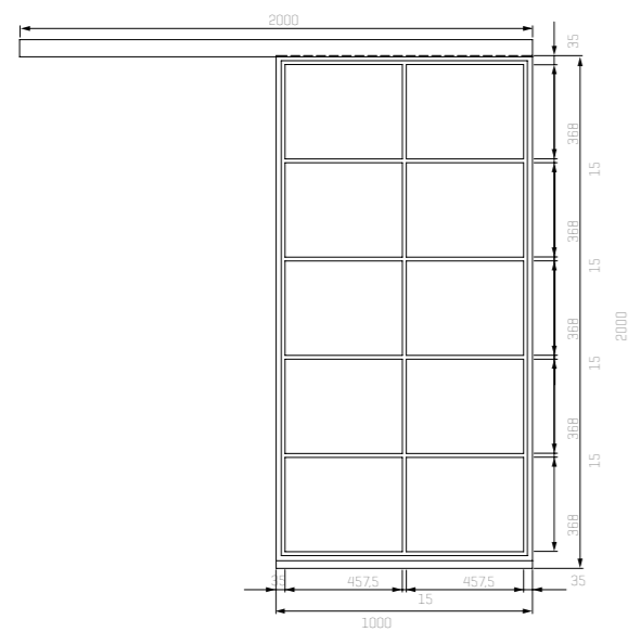
1-flüglige Stahl-Lofttür
