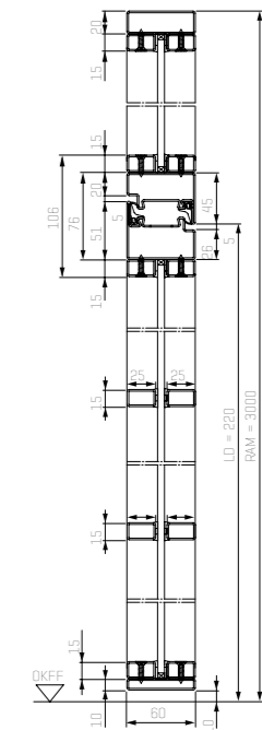
Vertikalschnitt 2-flügelige Stahl-Lofttür mit Oberlicht
