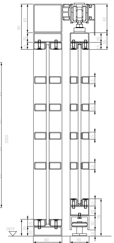
Vertikalschnitt 2-flüglige Stahl-Lofttür mit Seitenteilen
