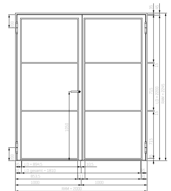
2-flüglige Stahl-Lofttür
