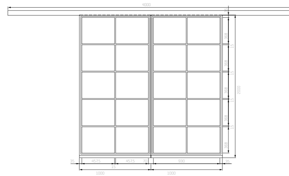
2-flüglige Stahl-Lofttür
