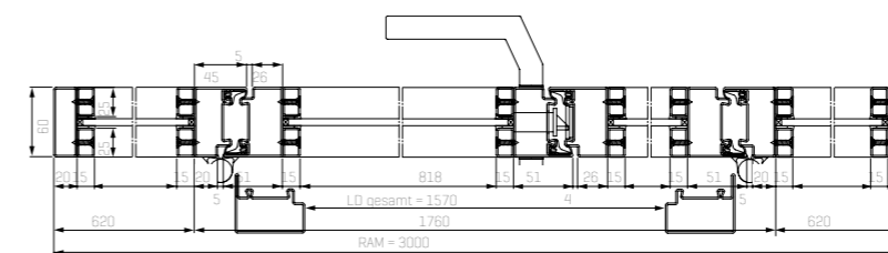
Horizontalschnitt 2-flügelige Stahl-Lofttür mit Seitenteilen
