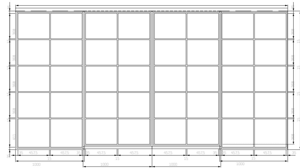
2-flüglige Stahl-Lofttür mit Seitenteilen
