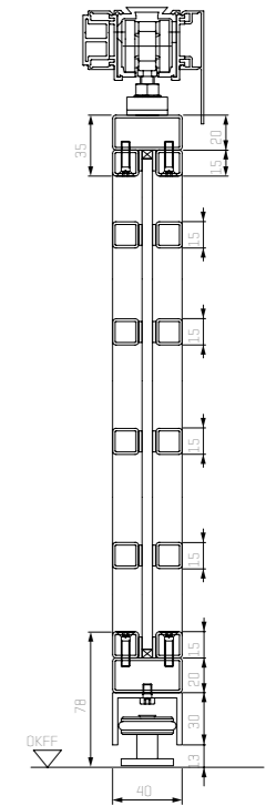
Vertikalschnitt 2-flüglige Stahl-Lofttür
