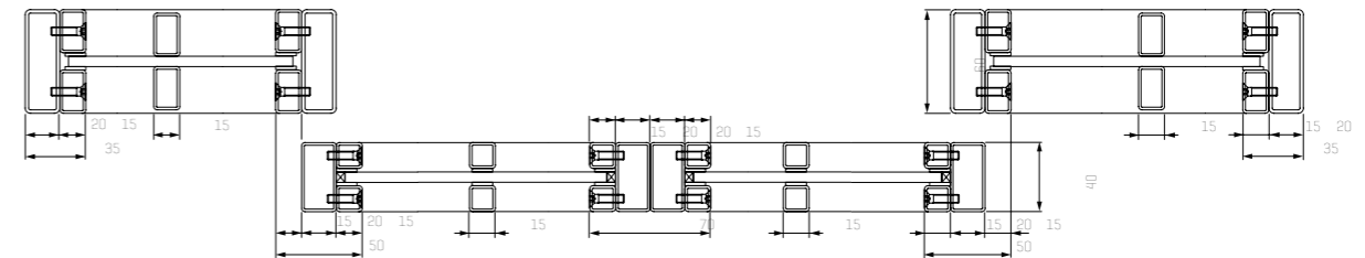
Horizontalschnitt 2-flüglige Stahl-Lofttür mit Seitenteilen
