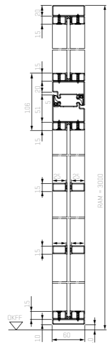
Vertikalschnitt 1-flügelige Stahl-Lofttür mit Oberlicht
