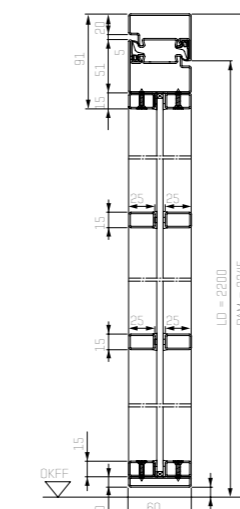
Vertikalschnitt 1-flüglige Stahl-Lofttür
